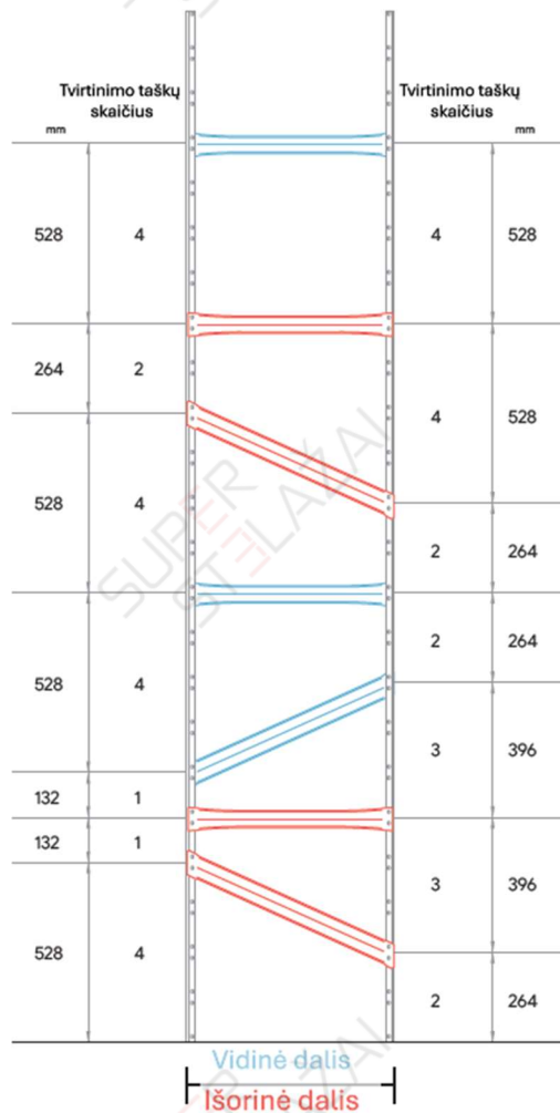
SUPER 1-2-3 H3000mm rėmas
