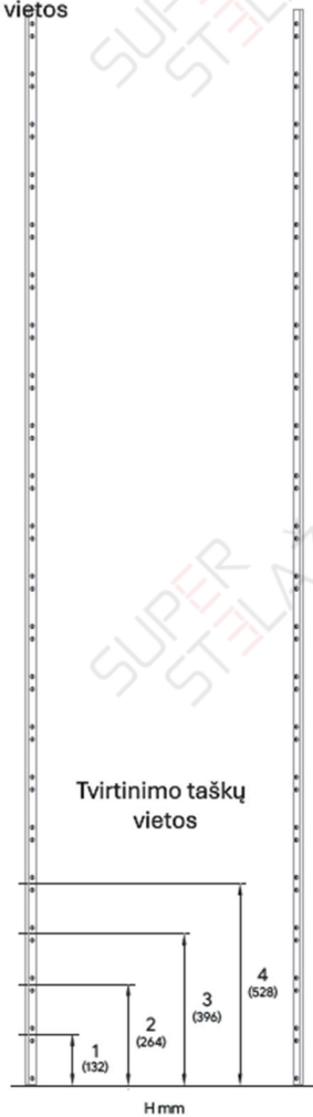
SUPER 1-2-3 Rėmo horizontalių ir diagonalių tvirtinimo taškų vietos
